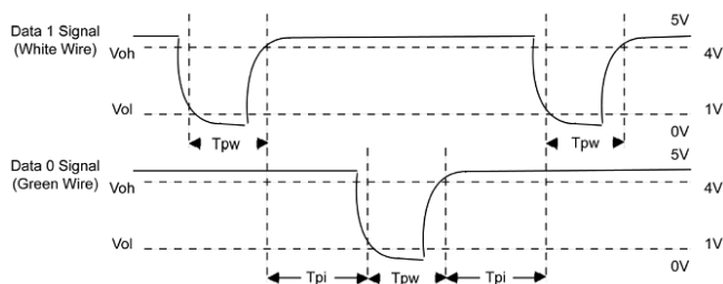
Рис.1: Диаграмма последовательности
